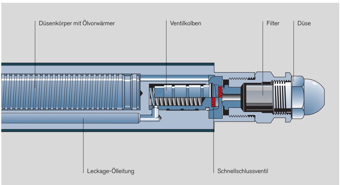
Das Weishaupt Düsenabschluss System verhindert ein Nachtropfen des Brennstoffes beim Anfahren und Abschalten des Brenners und reduziert zusätzlich Schadstoffemissionen
